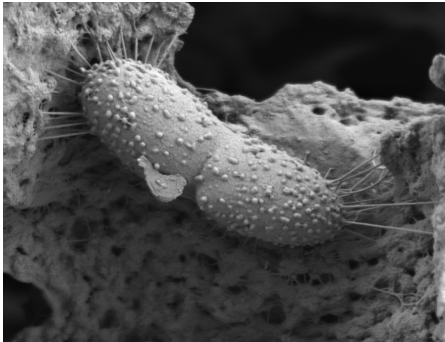
12C-Toluol, Innenseite, 09.05.07, 1,0kV, 5mm, 15000x
